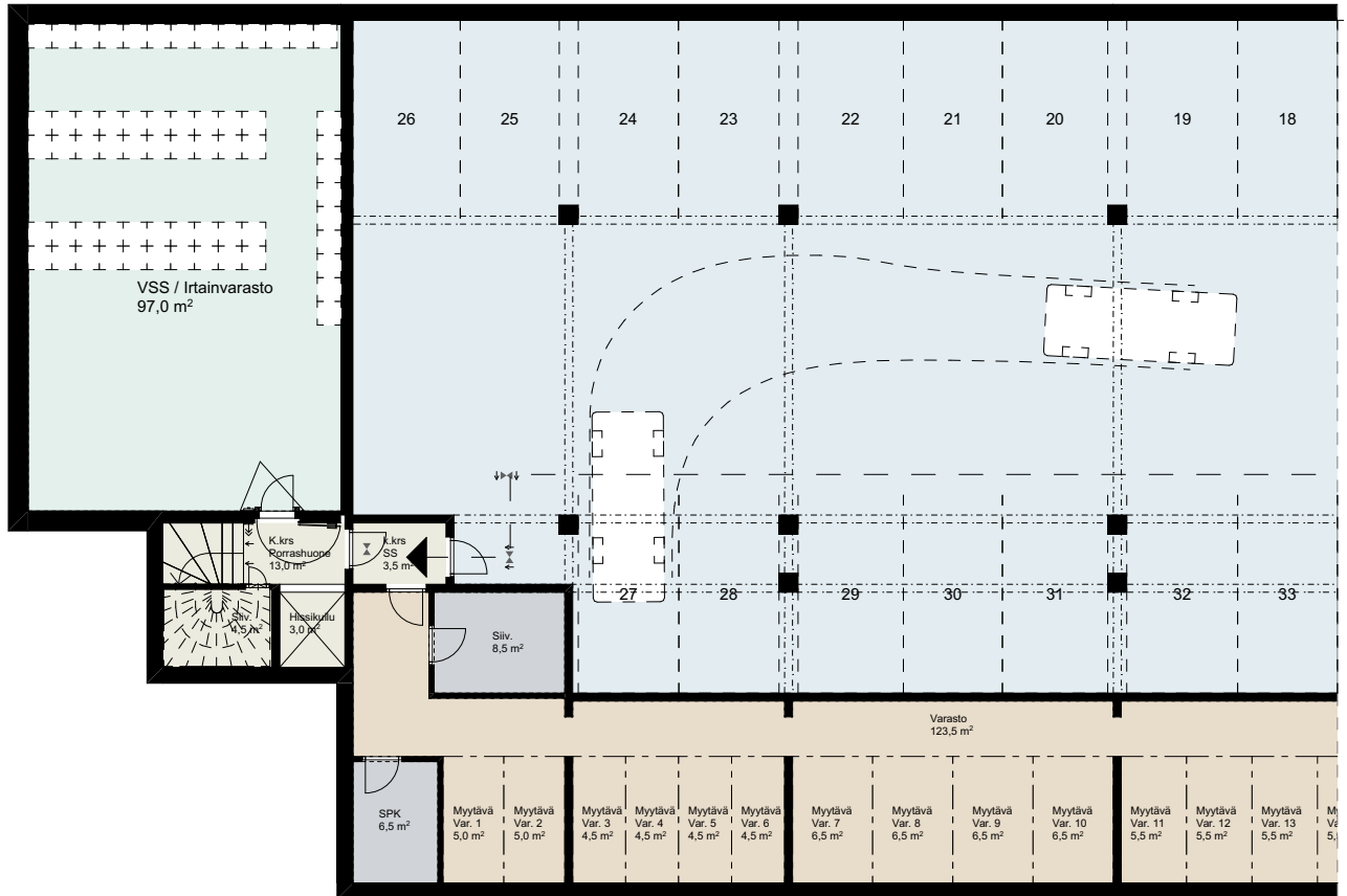
Talo A - K. krs
