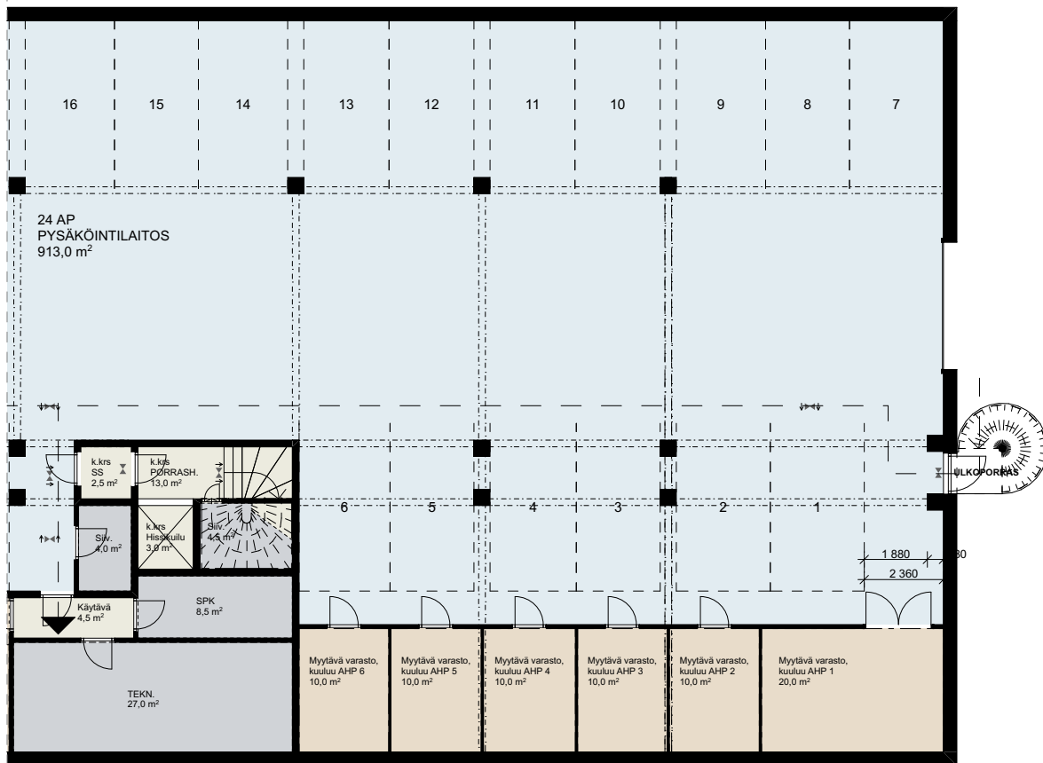
Talo B - K. krs
