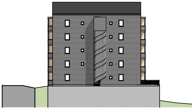
Julkisivu itään (Talo A)
